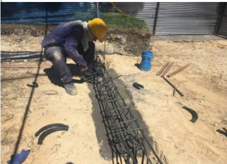
CONFORMACIÓN CANASTILLA PARA VIGAS DE CIMENTACIÓN JARDINERAS
