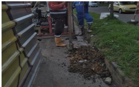
Perforación para instalación de instrumentación geotécnica
